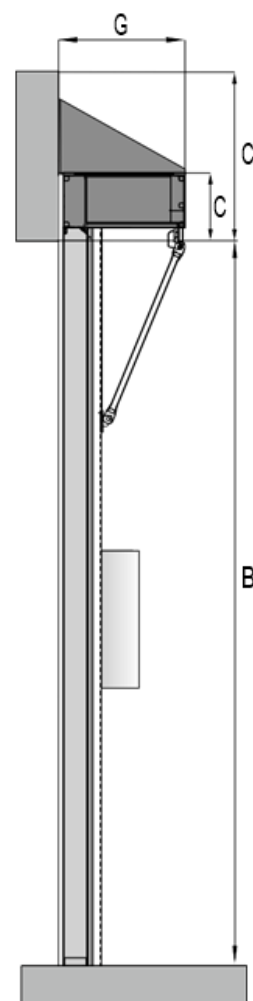
Przekrój pionowy
