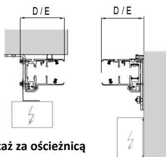
Przekrój poziomy
