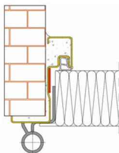
OŚCIEŻNICA NAROŻNA
