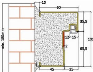
Wymiary ościeżnicy wewnętrznej przeciwpożarowej
